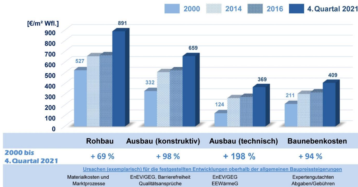
Abbildung 15: Entwicklung der Bauwerkskosten im Wohnungsneubau (ARGE-Kostenindex, Bezug Typengebäude MFH ) unter Berücksichtigung der Mehrwertsteuer, differenziert nach übergeordneten Leistungsbereichen unter Nennung der Baunebenkosten; Zeitraum: 1. Quartal 2000 bis 4. Quartal 2021; Kostenangaben in Euro je Quadratmeter Wohnfläche
