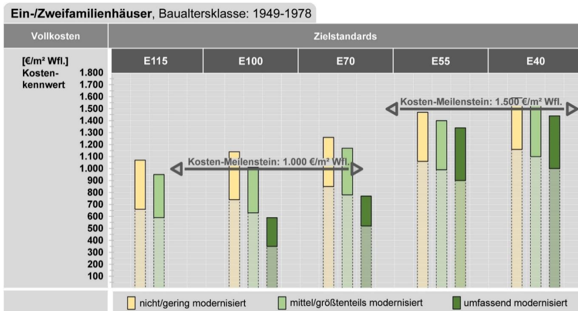
Abbildung 31: Darstellung der unterschiedlichen Kostenniveaus (Vollkosten) der energetischen Gebäudemoder- nisierung in Abhängigkeit zum Ausgangszustand und zum angestrebten energetischen Zielstandards, Ein-/ Zwei- familienhäuser der Baualtersklasse 1949-1978; Grundlage: Auswertung durchgeführter und abgerechneter Mo- dernisierungsvorhaben in Deutschland; Kostenstand: 3. Quartal 2021; Angaben in Form von spezifischen Kos- tenspannen in Euro je Quadratmeter Wohnfläche, inkl. Mehrwertsteuer (Bruttokosten)
