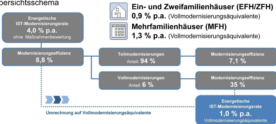
Abbildung 23: Übersichtsschema der energetischen IST-Modernisierungsrate in Verbindung mit der entsprechenden Modernisierungseffizienz inkl. Differenzierung von Teil- und Vollmodernisierungen, Bezug: Bestand an Wohngebäuden am 31.12.2020 (ohne Wohnheime)
