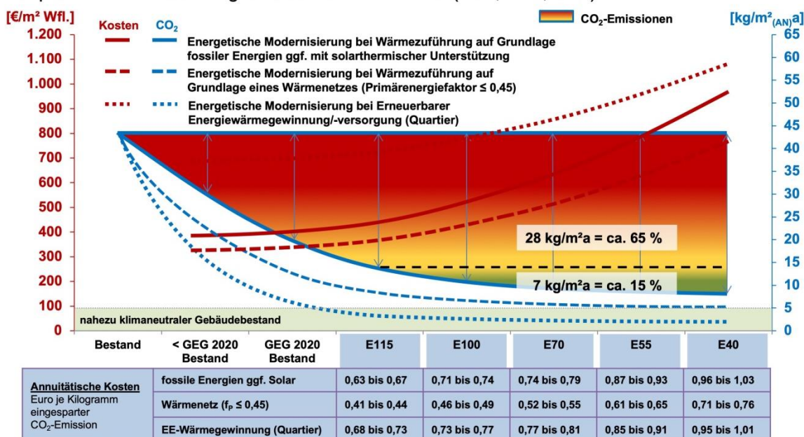
Abbildung 35: Trendanalyse – Kosten und CO 2 -Emissionen auf der Basis des tatsächlichen Energieverbrauchs am Beispiel der Geschosswohnungsbauten der 1950er bis 1970er Jahre für unterschiedliche energetische Modernisierungszustände. Die wirtschaftliche Vorteilhaftigkeit des „Effizienzhauses 115“ mit unterschiedlichen Qualitäten der Energieversorgung als Zielstandard für einen „nahezu klimaneutralen Gebäudebestand“ ist deutlich sichtbar.
