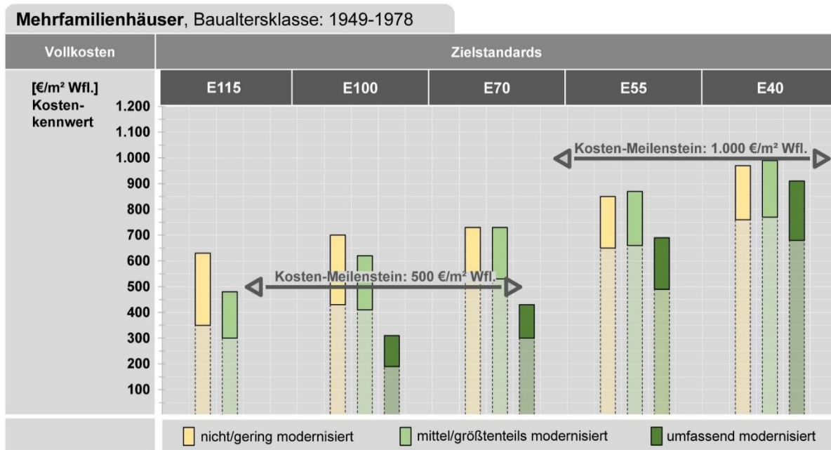
Abbildung 29: Darstellung der unterschiedlichen Kostenniveaus (Vollkosten) der energetischen Gebäudemodernisierung in Abhängigkeit zum Ausgangszustand und zum angestrebten energetischen Zielstandards, Mehrfamilienhäuser der Baualtersklasse 1949-1978; Grundlage: Auswertung durchgeführter und abgerechneter Modernisierungsvorhaben in Deutschland; Kostenstand: 3. Quartal 2021; Angaben in Form von spezifischen Kostenspannen in Euro je Quadratmeter Wohnfläche, inkl. Mehrwertsteuer (Bruttokosten)
