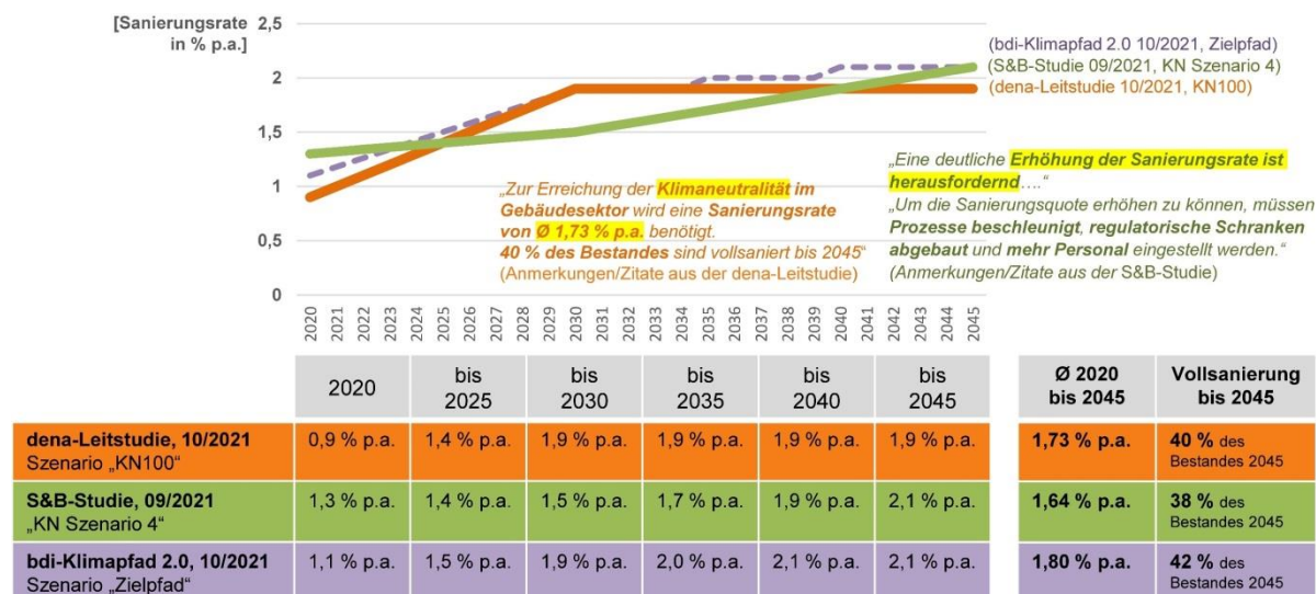
Abbildung 25: Vergleichsbetrachtung zur Entwicklung der Sanierungsrate bis 2045, Darstellung von Szenarien zur Entwicklung der übergeordneten Sanierungsrate aus aktuellen Sanierungsfahrplänen (Vollmodernisierungs-äquivalente) Quelle: Eigene Darstellung auf Basis dena-Leitstudie (10/2021), S&B-Studie (09/2021) und bdi-Klimapfad 2.0 (10/2021)
