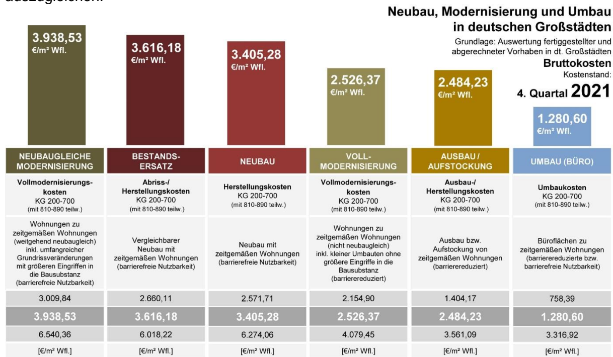
Abbildung 20: Baukosten-Vergleich realisierter Wohnungsbauvorhaben aus den Bereichen: (1.) Neubaugleiche Modernisierung mit Um- und Ausbau von Wohngebäuden der 1950er und 1960er Baujahre zu zeitgemäßen Wohnungen, (2.) Bestandsersatz von Wohngebäuden, (3.) Neubau von Wohngebäuden, (3.) Vollmodernisierung von Wohngebäuden, (4.) Ausbau von Dachgeschossen und Aufstockung von Wohngebäuden (5.) Umbau von Bürogebäuden bzw. Büroflächen zu zeitgemäßen Wohnungen. (Kostenstand: 4. Quartal 2021 - Kostengruppen 200-700 DIN 276)
